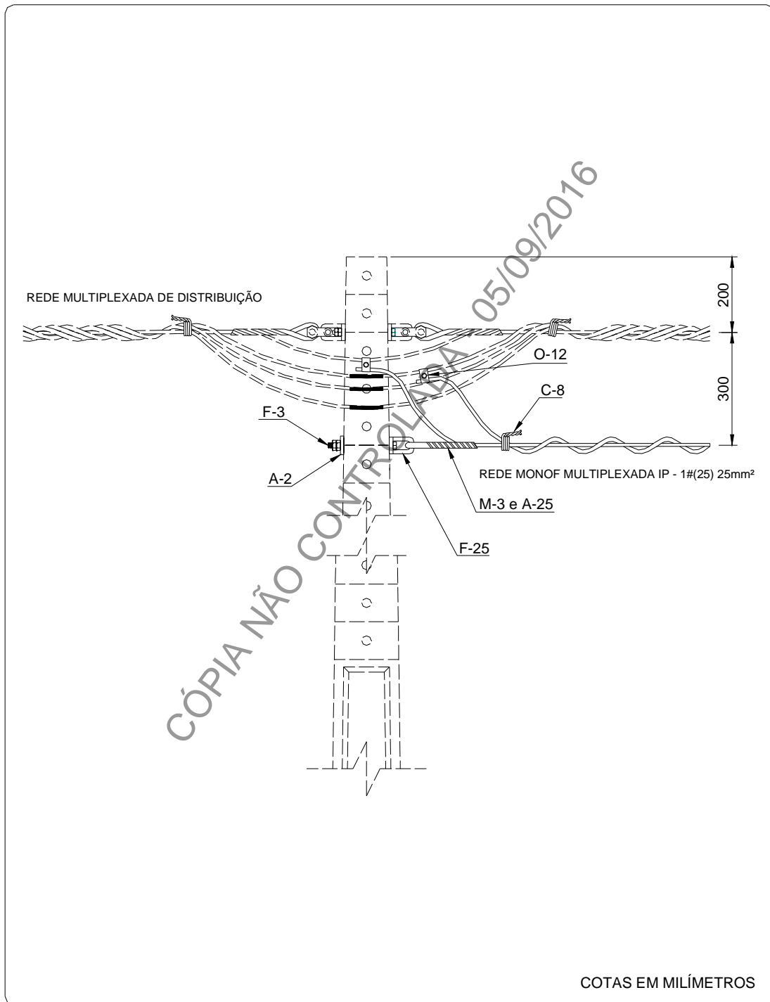
FIGURA 06 - ESTRUTURA IP-AC Estrutura de alimentação do circuito
